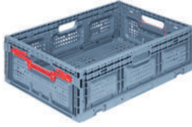
PG-6418 En/W Boy/L Yük/H Dış / Ext 400 x 600 x 185 mm İç / Int 362 x 576 x 176 mm Katlanmış Yükseklik 32 mm Folded Height 30 mm
