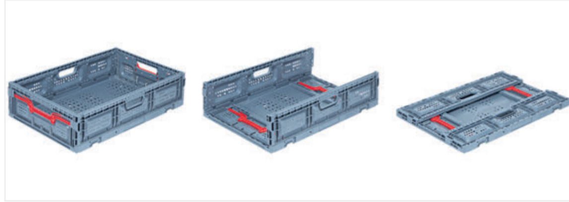
PG-6426 En/W Boy/L Yük/H Dış / Ext 400 x 600 x 259 mm İç / Int 376 x 576 x 251 mm Katlanmış Yükseklik 47 mm Folded Height 47 mm
