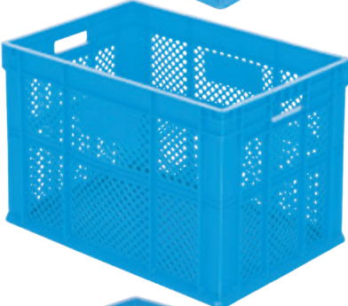
HP-4002 Kod / Code En/W Boy/L Yük/H Dış / Ext 400 x 600 x 400 mm İç / Int 365 x 565 x 386 mm
