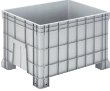
K-330 En/W Boy/L Yük/H Dış / Ext 670 x 930 x 625 mm İç / İnt 620 x 890 x 520 mm
