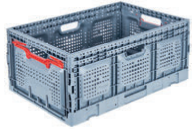
PG-6426 En/W Boy/L Yük/H Dış / Ext 400 x 600 x 259 mm İç / Int 376 x 576 x 251 mm Katlanmış Yükseklik 47 mm Folded Height 47 mm
